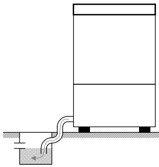
Свободный слив
